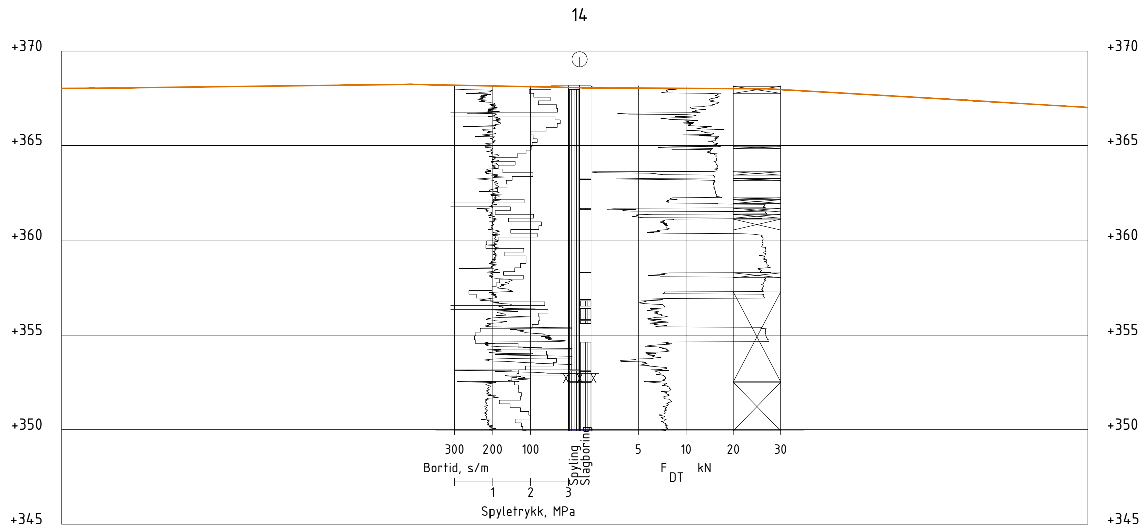
Profil F-F
